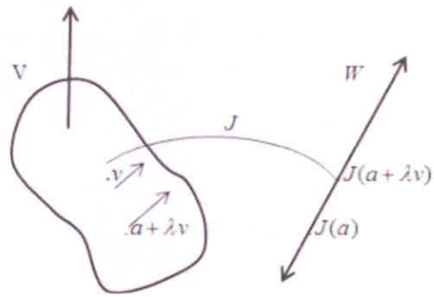
Figura C.3: Derivada direccional.
