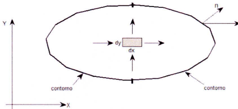
Figura 1.5: Dominio bidimensional.
