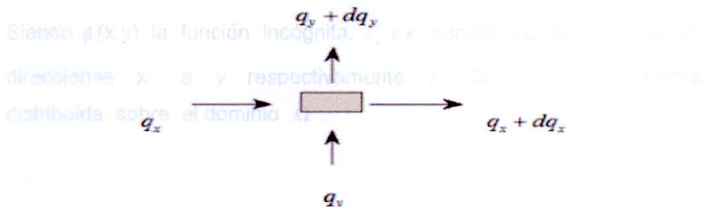
Figura 1.6: Balance de flujos de calor en un dominio bidimensional.
